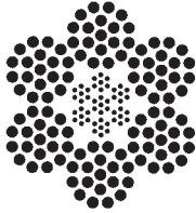
6x19 IWRC
